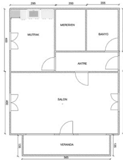
62,5m² Dupleks Ev Zemin Kat Planı
