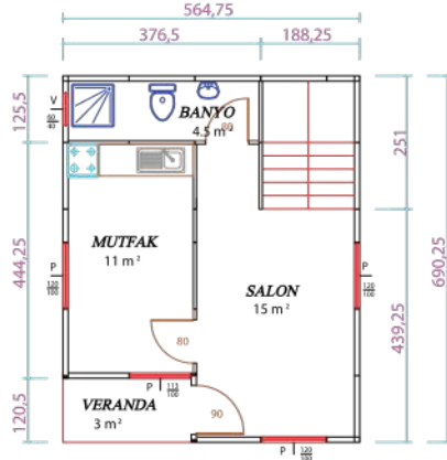
33m² Dupleks Ev Zemin Kat Planı
