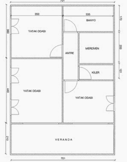
52m² Dupleks Ev Üst Kat Planı
