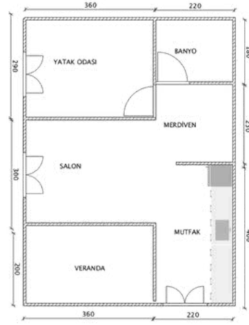
46m 2 Dupleks Ev Zemin Kat Planı
