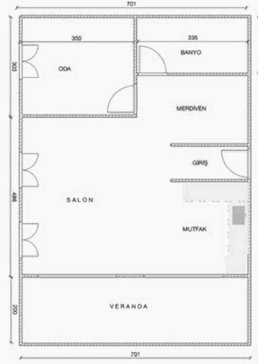
52m² Dupleks Ev Zemin Kat Planı
