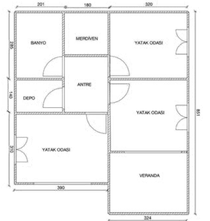
57m² Dupleks Ev Üst Kat Planı
