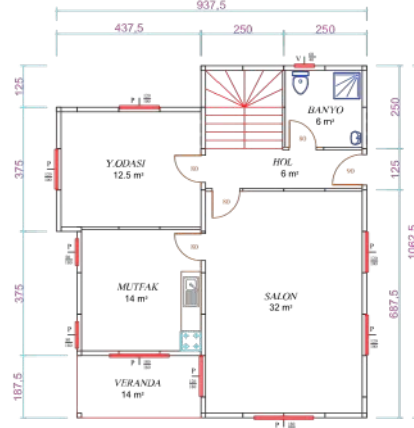
90m 2 Dupleks Ev Zemin Katı Planı
