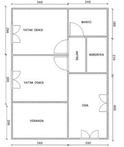
46m 2 Dupleks Ev Üstü Kat Planı
