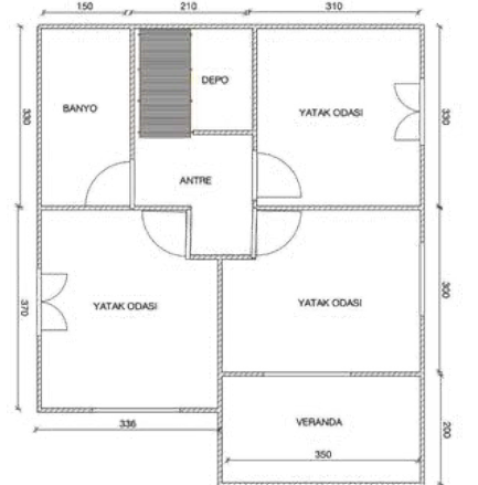
57m 2 Dupleks Ev Üstü Kat Planı
