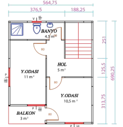
34m² Dupleks Ev Üst Kat Planı
