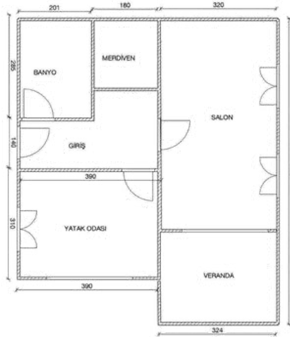
57m² Dupleks Ev Zemin Kat Planı
