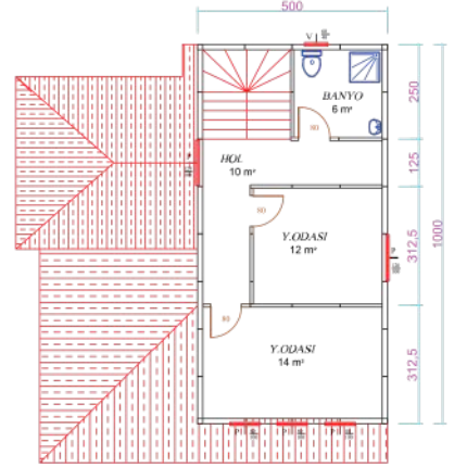
50m 2 Dupleks Ev Üst Katı Planı
