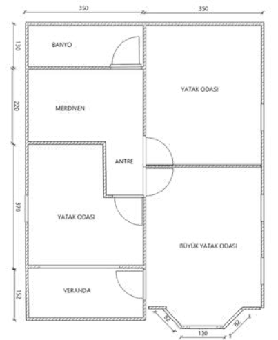
60m 2 Dupleks Ev Üst Katı Planı
