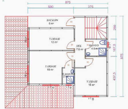
70m 2 Dupleks Ev Üst Katı Planı
