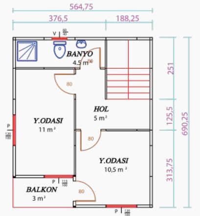
34m 2 Dupleks Ev Üstü Kat Planı
