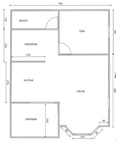
60m 2 Dupleks Ev Zemin Katı Planı
